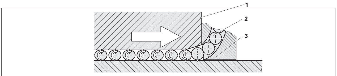
1) Guides à billes 2) Bille 3) Rail à billes
