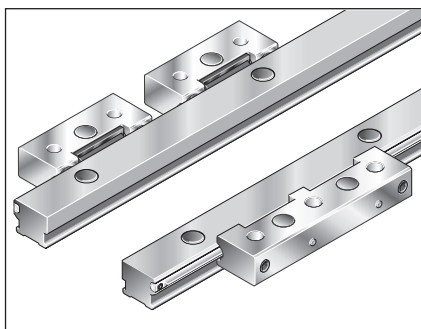
Cassettes simples, Cassettes doubles Sur deux demi-rails
