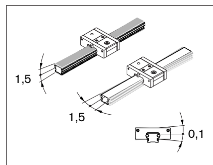
Guides Super Pour toutes les surfaces de montage irrégulières et pour tous les autres défauts d'alignement:
