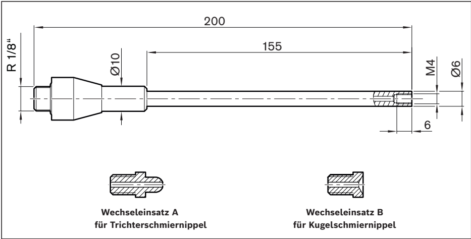
Düsenrohr für Handfettpressen. Zur Schmierung von Trichter- und Kugelschmiernippel für Kugelwagen Größe 15 und 20. Lieferumfang: 1 x Düsenrohr 1 x Wechseleinsatz A für Trichterschmiernippel 1 x Wechseleinsatz B für Kugelschmiernippel
