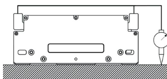
Ebenheit: 20 \mu\text{m} / 500 mm
