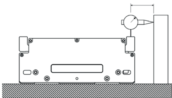
Geradheit: 10 \mu\text{m} / 500 mm
