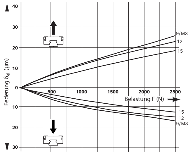
Führungswagen Breit Lang R0441
