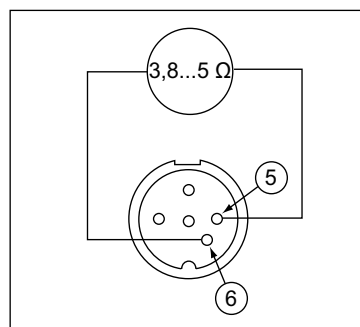
Connecteur i-TOOL
