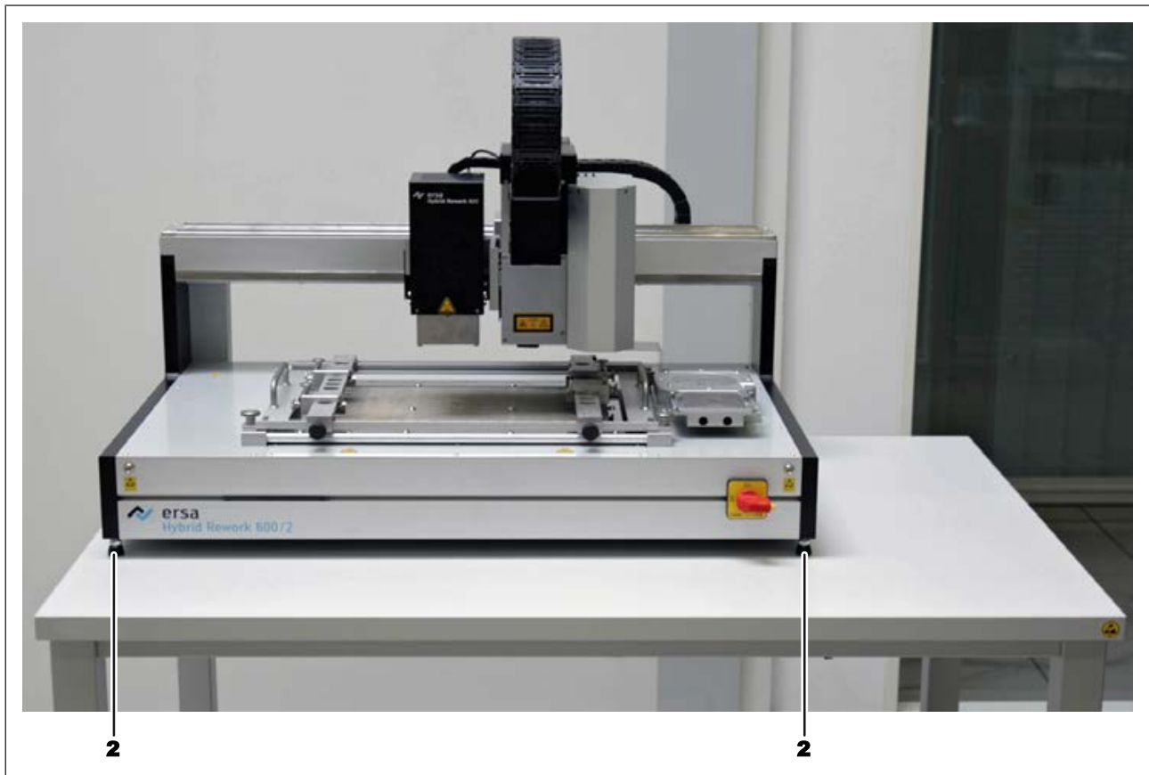
Abb. 6: HR 600/2 aufstellen
