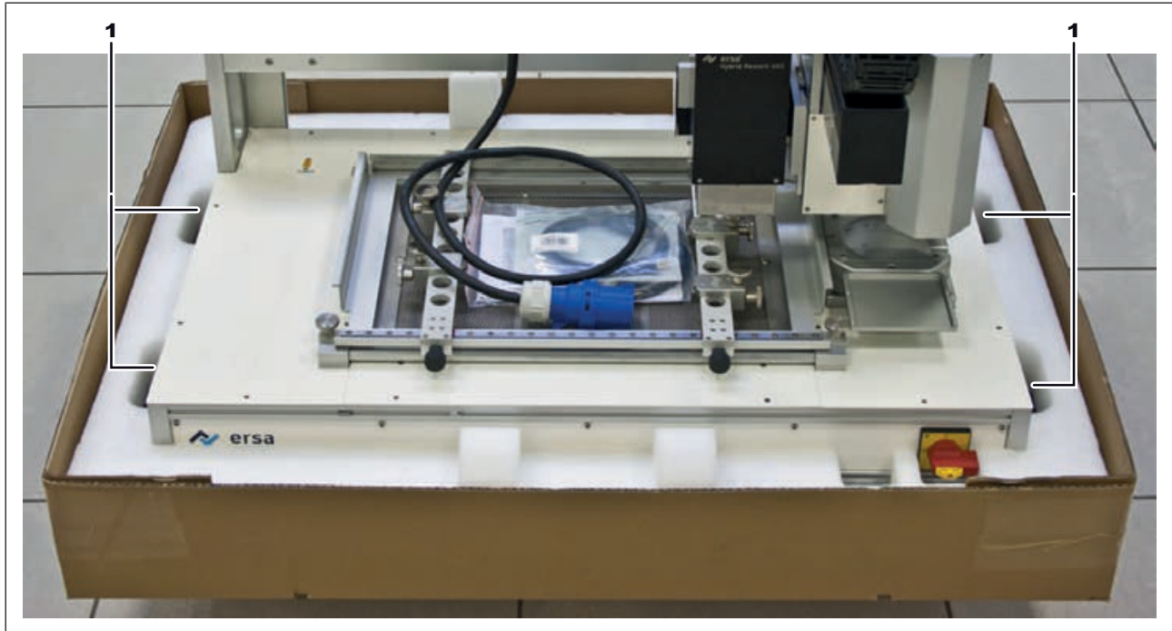
Abb. 5: Die Anhebepunkte
