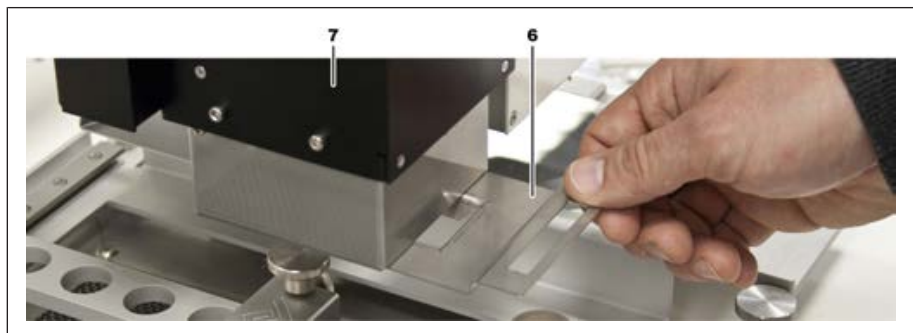
Abb. 9: Luftleitblech einschieben
