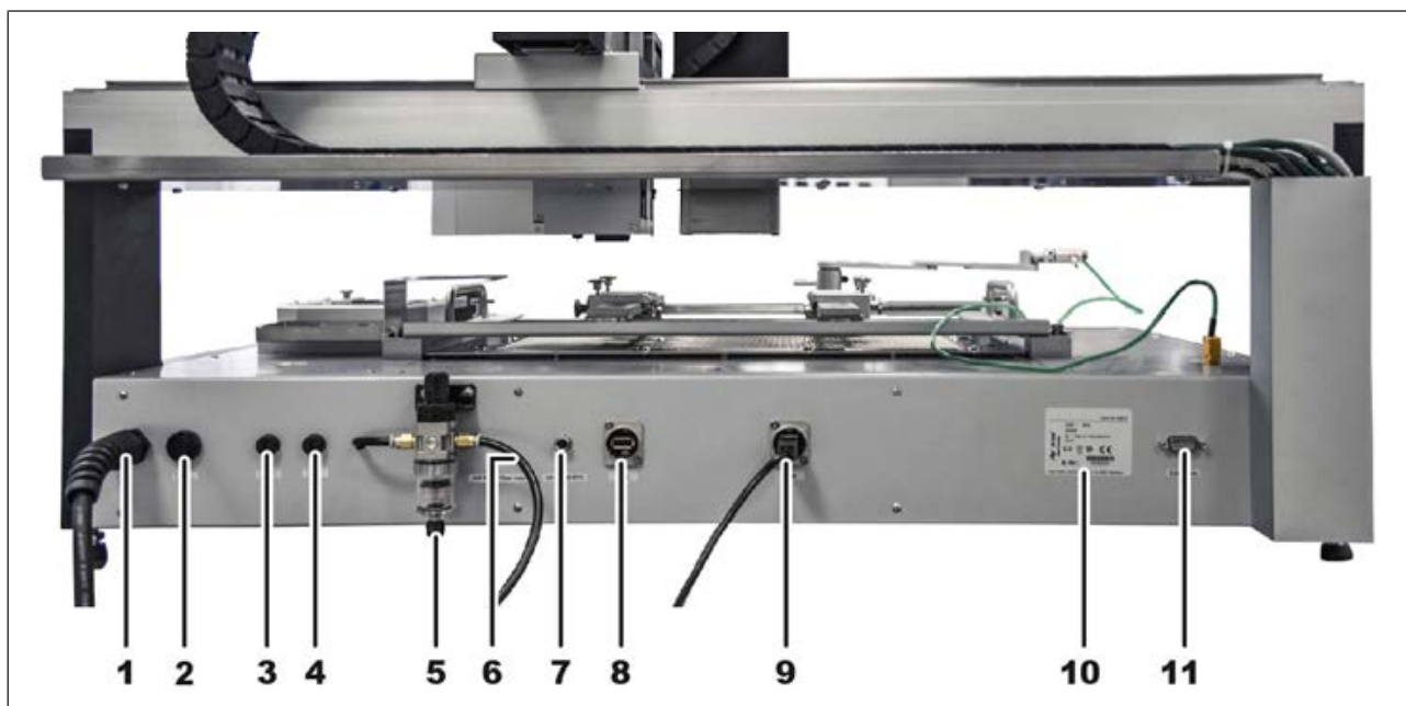
Abb. 7: Die Rückseite des HR 600/2
