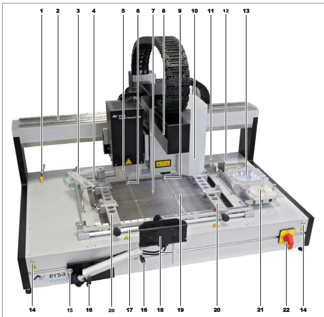
Abb. 12: Übersicht der Maschinenteile
