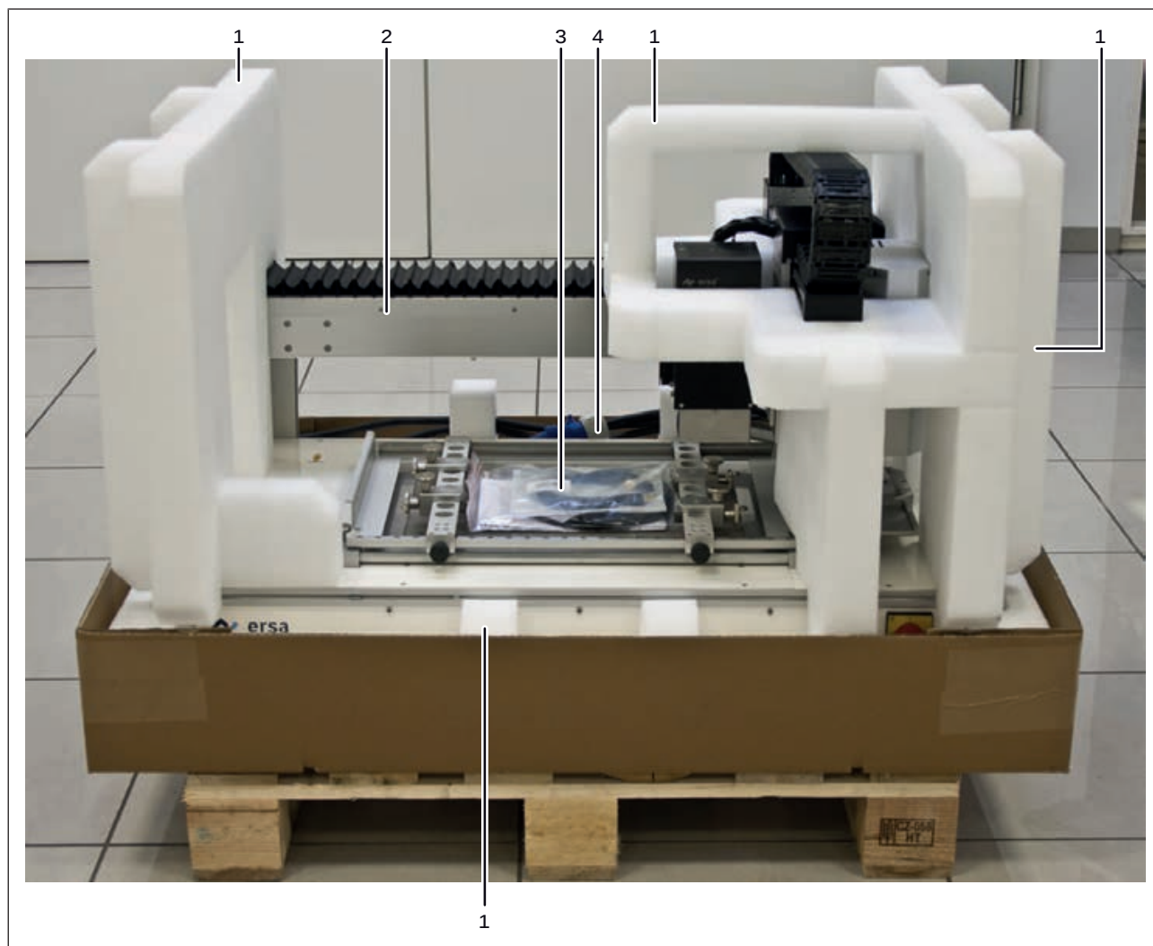
Abb. 4: Geöffnete Verpackung
