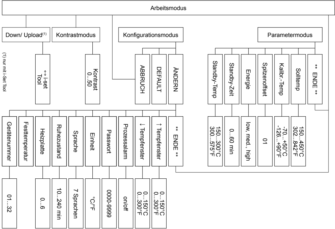
Funktionsübersicht i-CON 1
