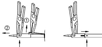
Soltar el gancho elástico de la ranura (1) y estrar de la punta con unas tenazas de boca plana (2).
