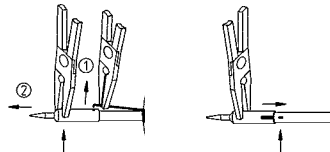
Verende klem van de soldeerpunthouder heffen (1) en punten met een platte tang verwijderen (2).
