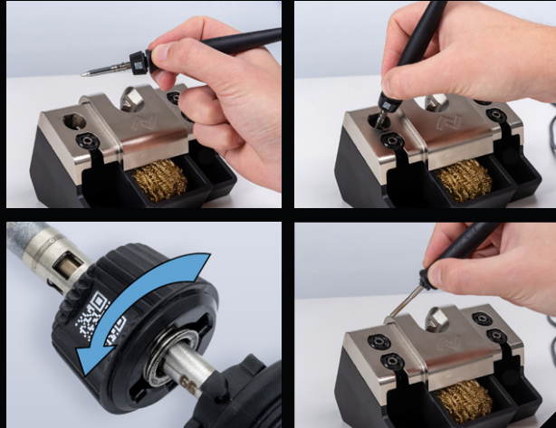
Changement de panne breveté directement dans le support
