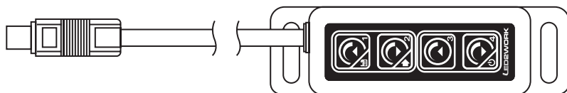
SYSTEMLED SurfaceOne Bedienelement mit 5m Anschlussleitung
