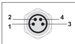
Diagrama del conector M8
