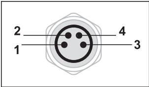
Disegno schematico connettore M8
