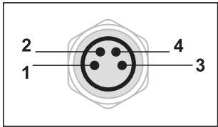
Schéma du connecteur M8
