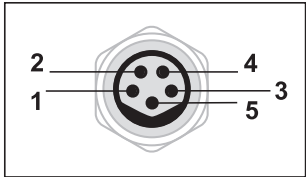
Schéma du connecteur M8
