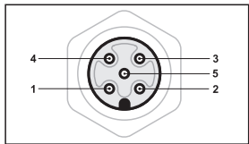
Diagrama del conector M12
