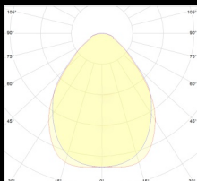
Lichtverteilung
