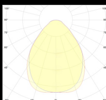
Lichtverteilung
