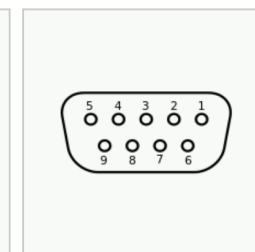
DE-9 1 9-pol Buchse (weiblich)
