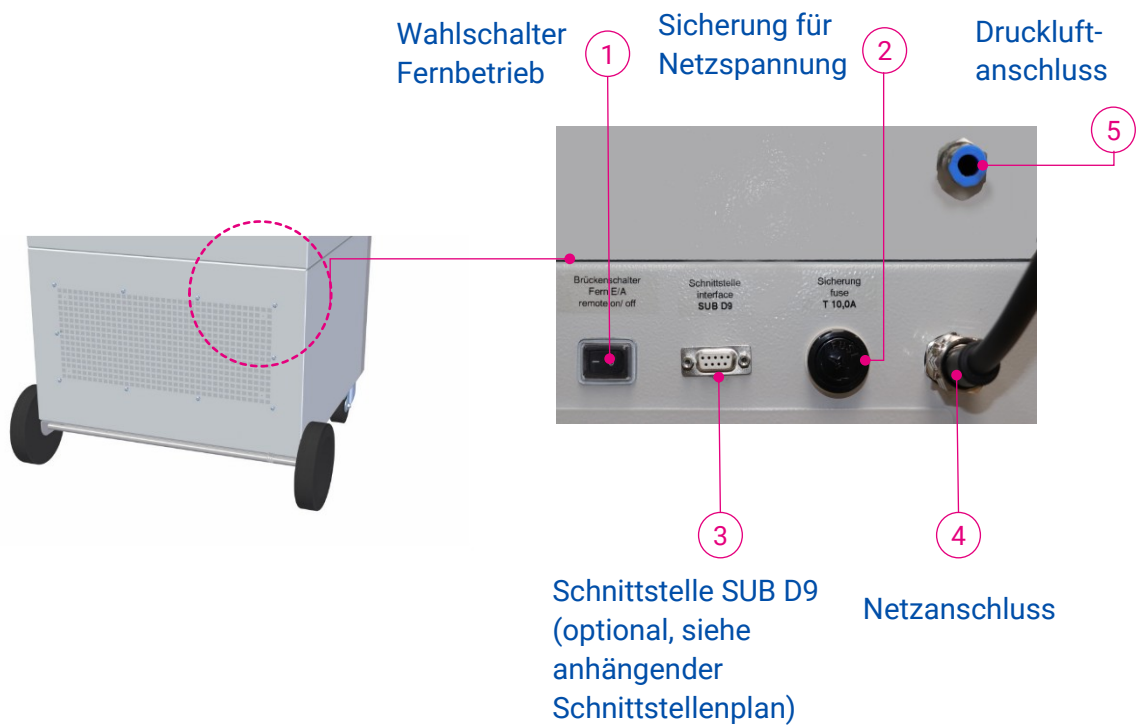
Abbildung 2: rückseitige Schnittstellen
