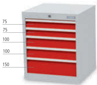
▪ 5 x Schublade
