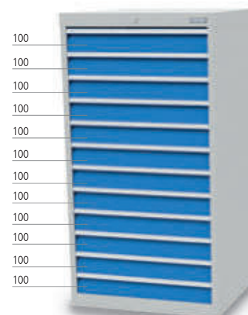
■ 12 x Schublade
