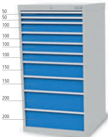
■ 10 x Schublade
