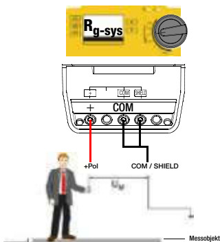
Messung: R_{G\text{-system}} Personenableitwiderstand (Mensch/Schuhe/Boden) zu Schutzerde
