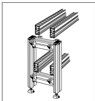
SZ2/E, SZ2/E-H, SZ2/T, SZ2/T-H, SZ2/U, SZ2/U-H Leg Sets 8-1 to 8-4
