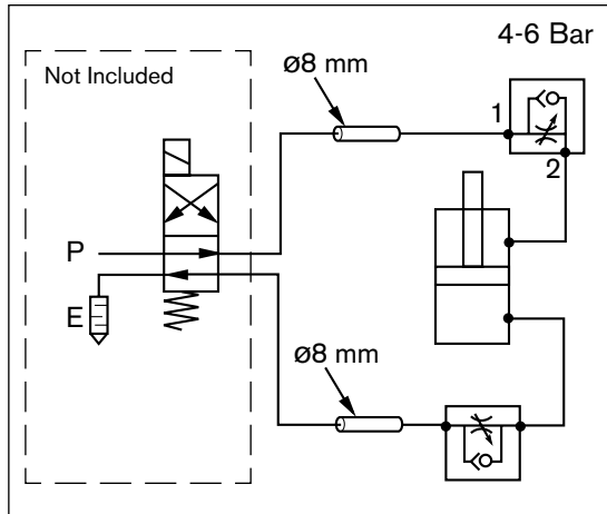
Pneumatic diagram for HP2, HP2/E, HP2/K, HD2/E
