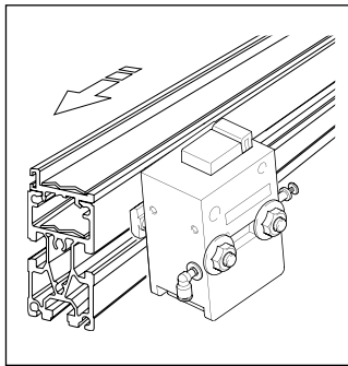
VE2, VE2/L, VE2/M Standard Stop Gates 15-1
